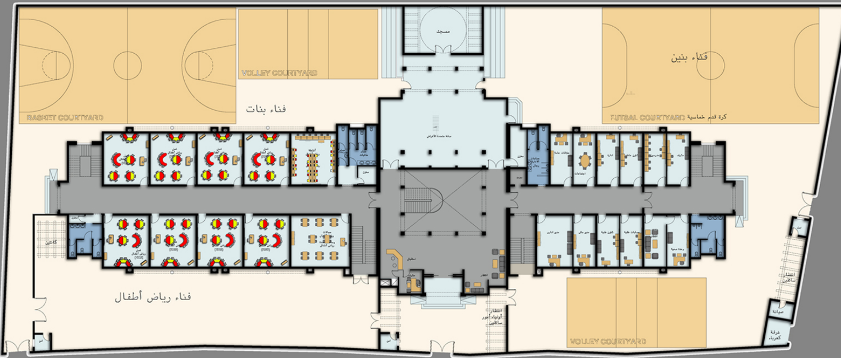
مسقط افقى للدور الأرضي
